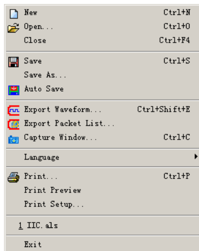
Fig 3-2: File menu.
